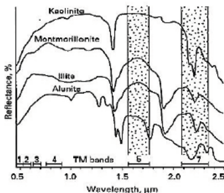
شکل ۱. نمودار طیف بازتابش بعضی از کانی‌های هیدروکسل‌دار و محدوده باندهای ۵ و ۷ سنجنده ETM +
